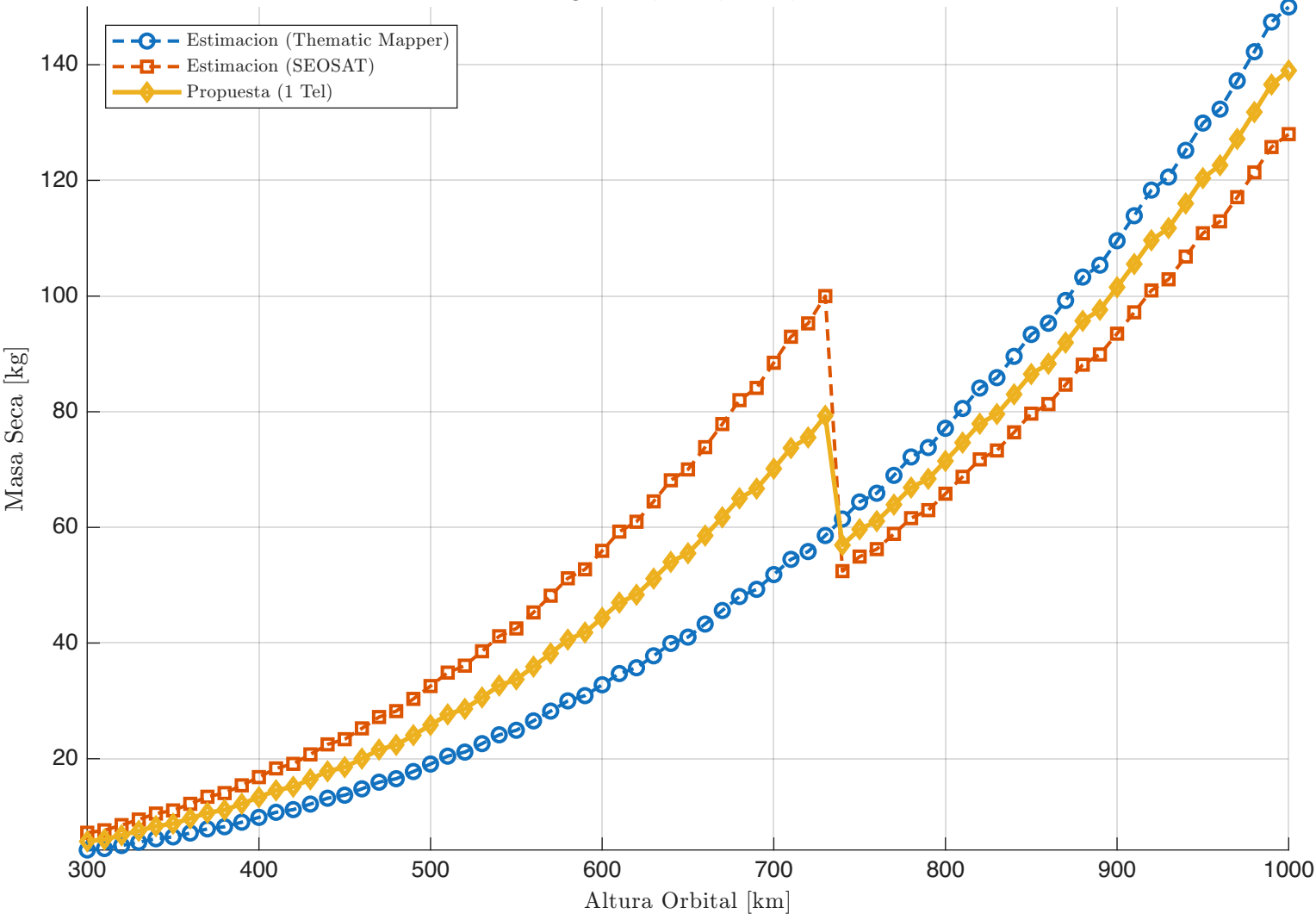
Comparativa de Masa Seca vs. Altura Config: 2 Sat, 1 Tel, Det 2, TMA
